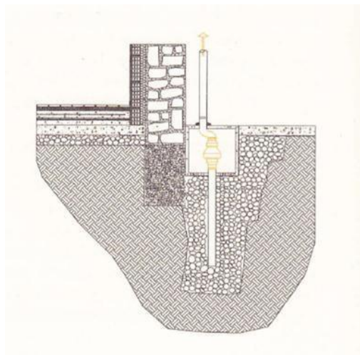
Figura 60: Schema di pozzetto d'aspirazione
