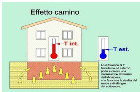
Figura 6: Effetto camino
