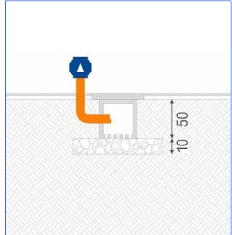
Figura 56: prevenzione nuova edificazione BONIFICA EDILIZIA ESISTENTE: TIPOLOGIE DI POZZETTI E DI CANALIZZAZIONI DI ASPIRAZIONE
